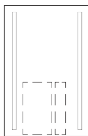
Finoflex® Spiegelmodul mit 2 Leuchten Nr. FF-662 mit 1 Leuchte Nr. FF-661 ohne Leuchte Nr. FF-660 H 1000 mm B 650 mm T 170 mm H Leuchtfeld 900 mm (ohne Zubehör)
